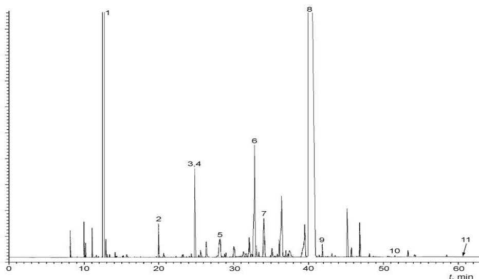
شکل الف-۲-۲- نمونه کروماتوگرام گونه چینی ۶۰٪، به دست آمده از ستون قطبی
