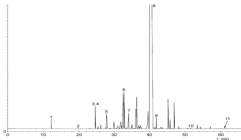
شکل الف-۱-۲-نمونه کروماتوگرام گونه چینی ۸۰٪، به دست آمده از ستون قطبی
