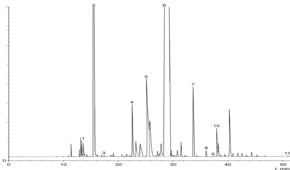
شکل الف-۲-۱- نمونه کروماتوگرام گونه چینی ۶۰٪، به دست آمده از ستون غیرقطبی
