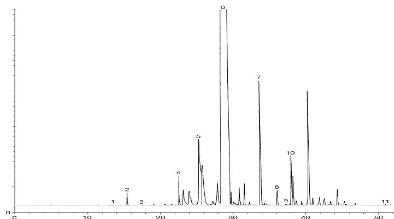
شکل الف - ۱-۱- نمونه کروماتوگرام گونه چینی ۸۰٪، به دست آمده از ستون غیرقطبی
